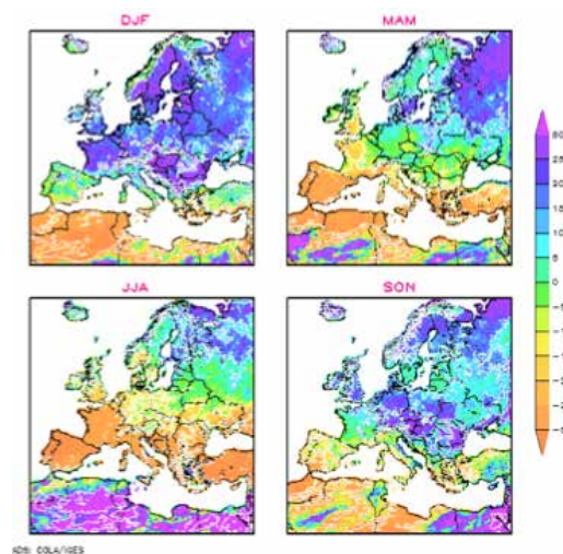
rechts Veränderung der Niederschläge in % für Winter, Frühling, Sommer und Herbst für die ferne Zukunft 2071-2100 im Vergleich zu 1961-1990 (A1B Szenario).
