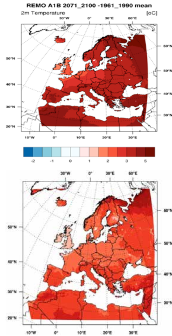
rechts Veränderungen der Temperatur [°C] in 2 m für Emissionsszenarien A1B und RCP4.5 (2071-2100 im Vergleich zu 1961-1990).
